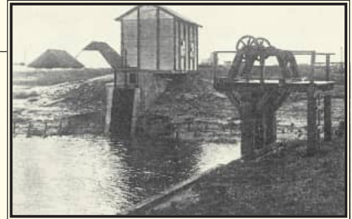
Vista parcial de la instalación con la esclusa y la casa de máquinas. Abajo, vista del dique y de las esclusas en diversas alturas, para hacer pasar el agua del mar de un estanque a otro.
